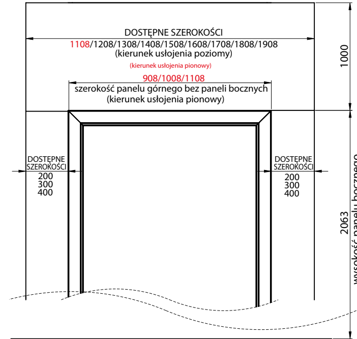
PANEL GÓRNY – OŚCIEŻNICA STAŁA DO DRZWI SOLLER, SELVA
