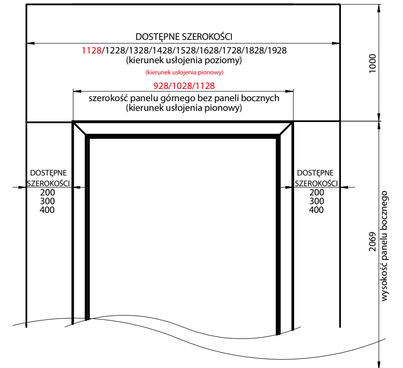
PANEL GÓRNY – OŚCIEŻNICA STAŁA DO DRZWI MAXUS RC2
